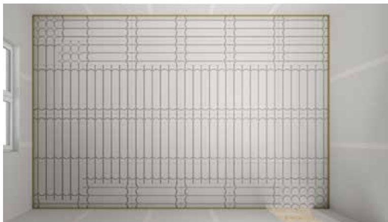
Instalační schéma se dvěma topnými okruhy.
